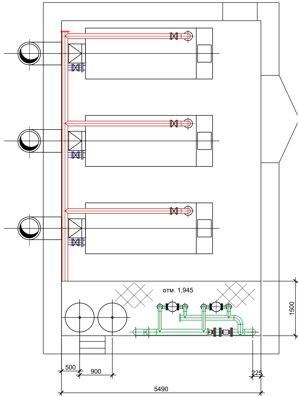
План на отм. 1,945
